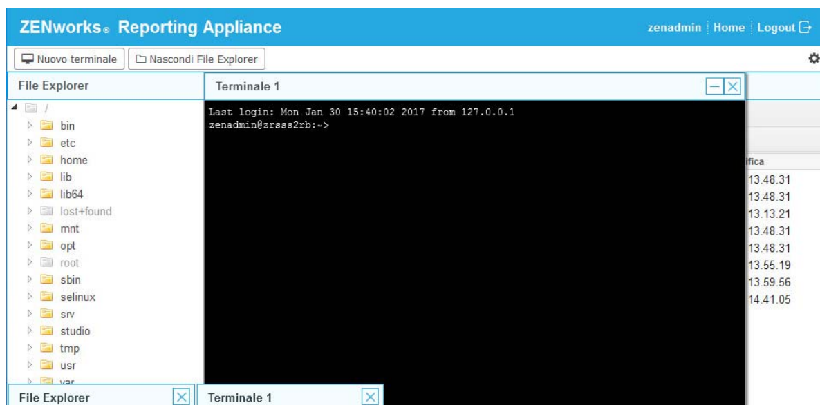
Figura 6-4 Terminale
